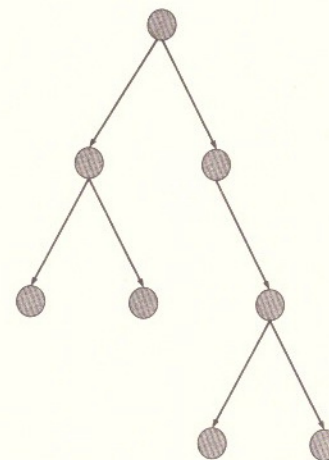
Фиг. 8. Йерархична мрежа – ориентиран двуделен граф
